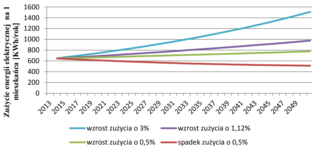
Rys. 9. Progniza jednostkowego zużycia energii elektrycznej dla Gminy Nowa Karczma do roku 2050 Źródło: Opracowanie własne na podstawie danych GUS
