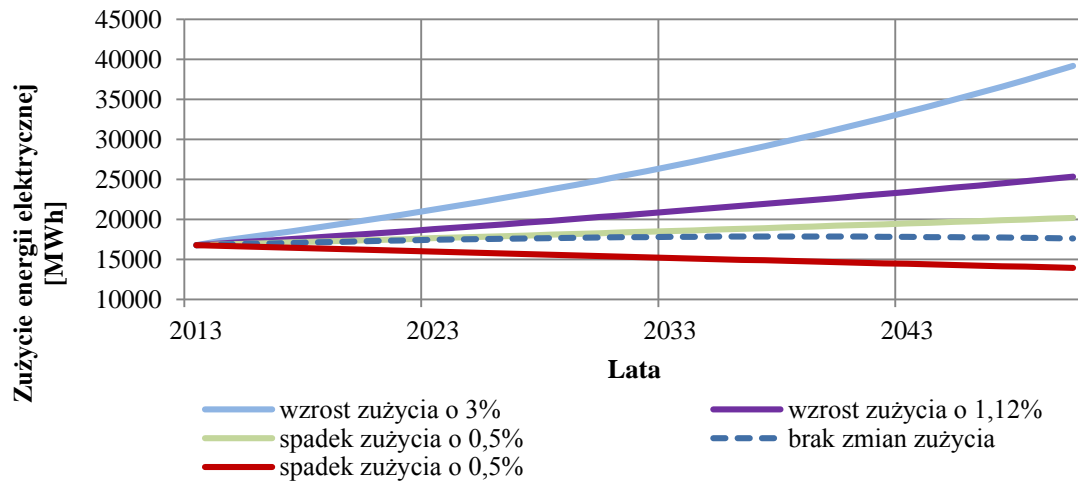
Rys. 12. Progniza całkowitego zużycia energii elektrycznej dla Gminy Stara Kiszewa do roku 2050 Źródło: Opracowanie własne na podstawie danych GUS
