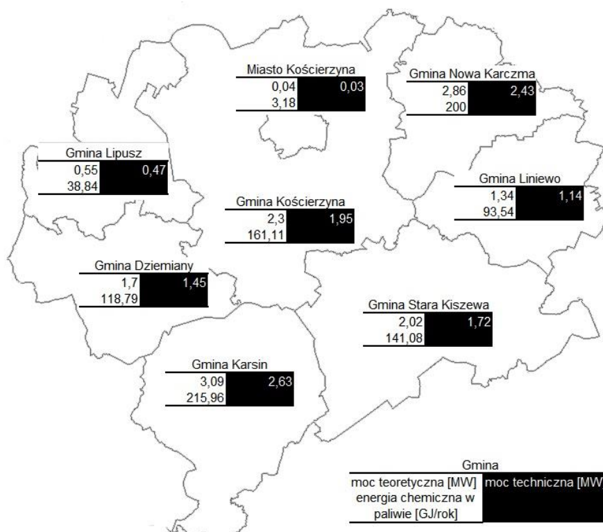
Rys. 38. Potencjał teoretyczny oraz techniczny biogazu rolniczego z produkcji rolniczej
