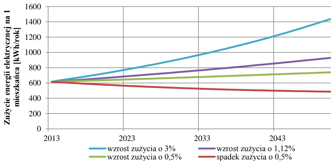
Rys. 13. Progniza jednostkowego zużycia energii elektrycznej dla Gminy Stara Kiszewa do roku 2050 Źródło: Opracowanie własne na podstawie danych GUS
