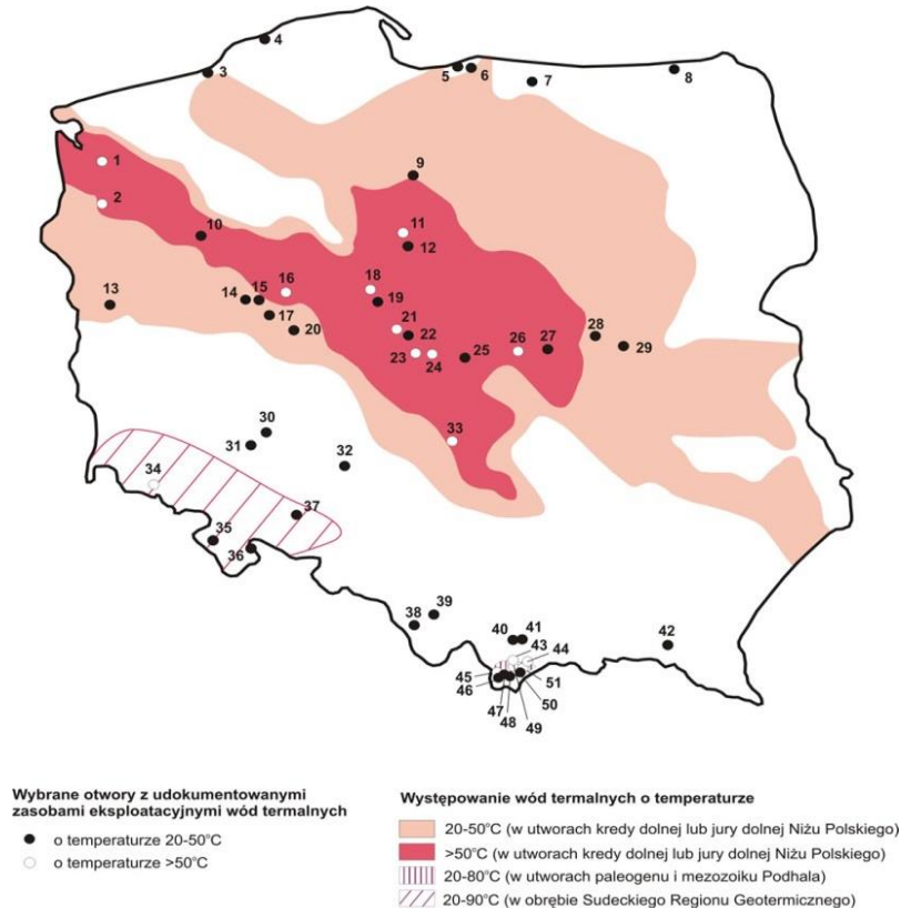
Rys. 60. Temperatura zbiornika Dolnej Jury Niziny Polskiej Źródło: www.mos.gov.pl
